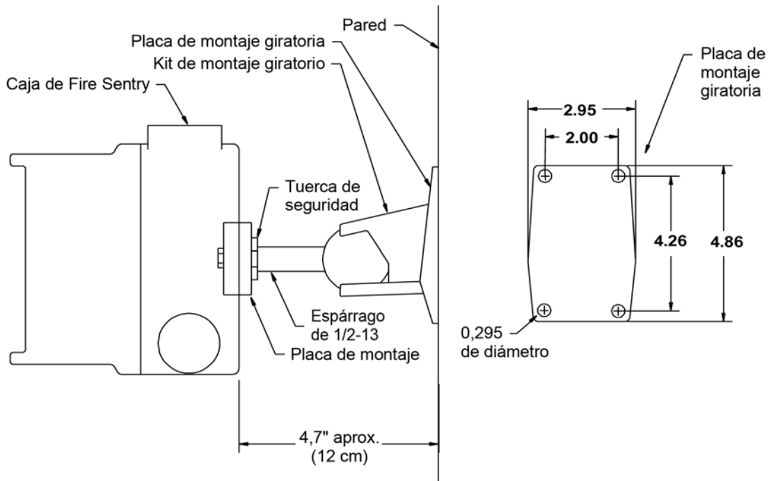
Figura 4: Kit de montaje giratorio modelo SM2
