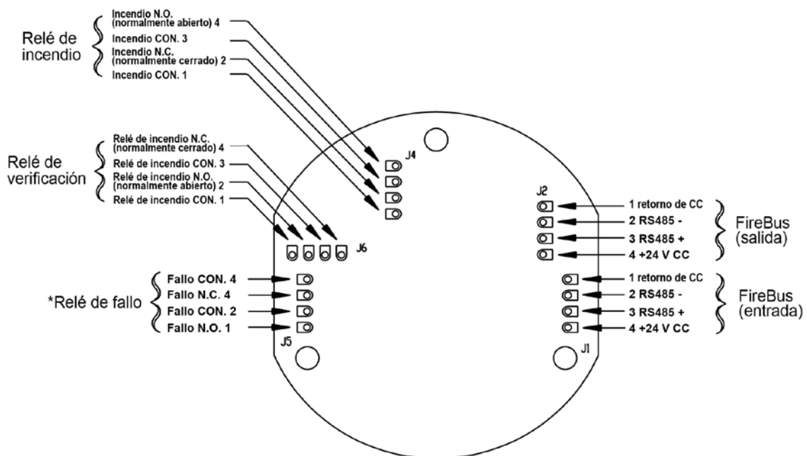
Figura 2: Cableado del detector modelo SS4-AS/-AS2 (vista trasera del módulo del detector SS4-AS/-AS2)
