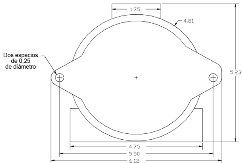
Figura 8: Caja del detector modelo SS4-AS/-AS2, vista trasera
