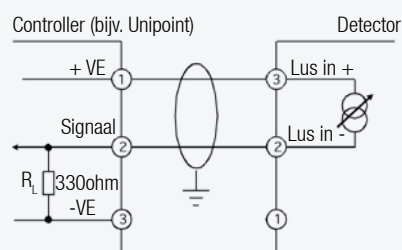
Typische giftige detectoraansluitingen (2 draads 4-20mA Ius)
