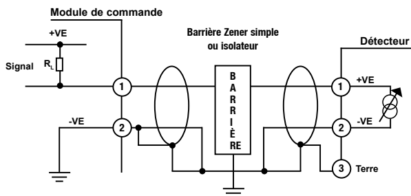
Schéma de barrière simple
