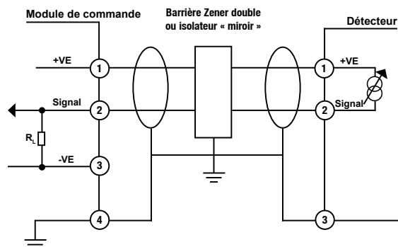
Schéma de barrière double
